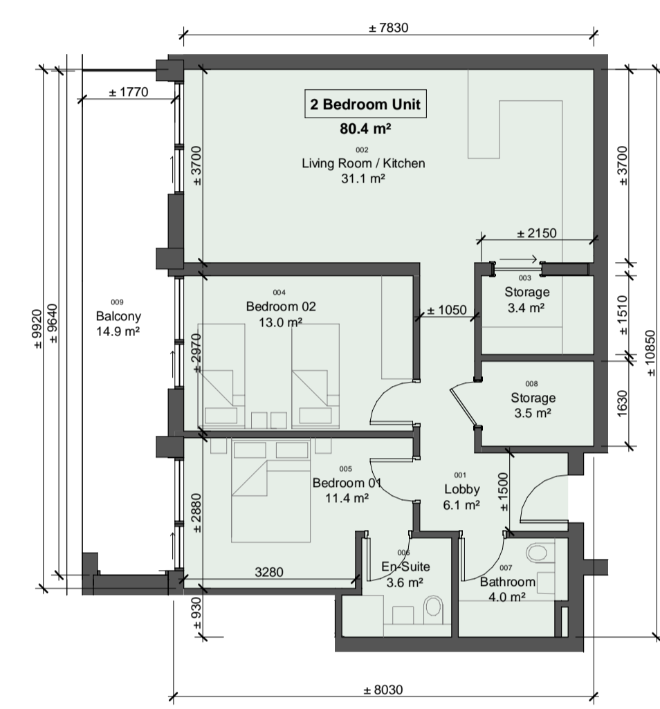
7 Unit Type 2BR-A-2 scale 1 : 100
