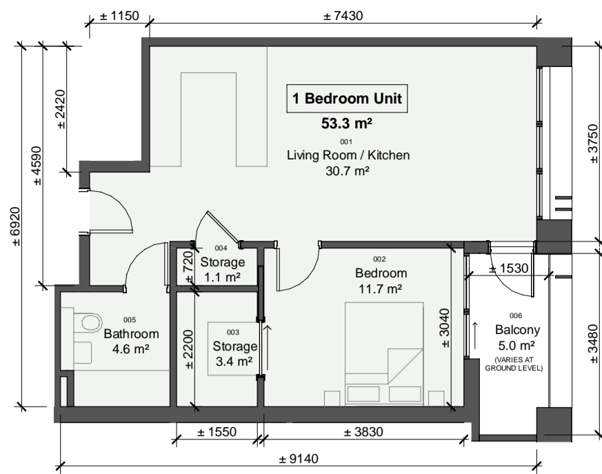
2 Unit Type 1BR-A-2 scale 1 : 100
